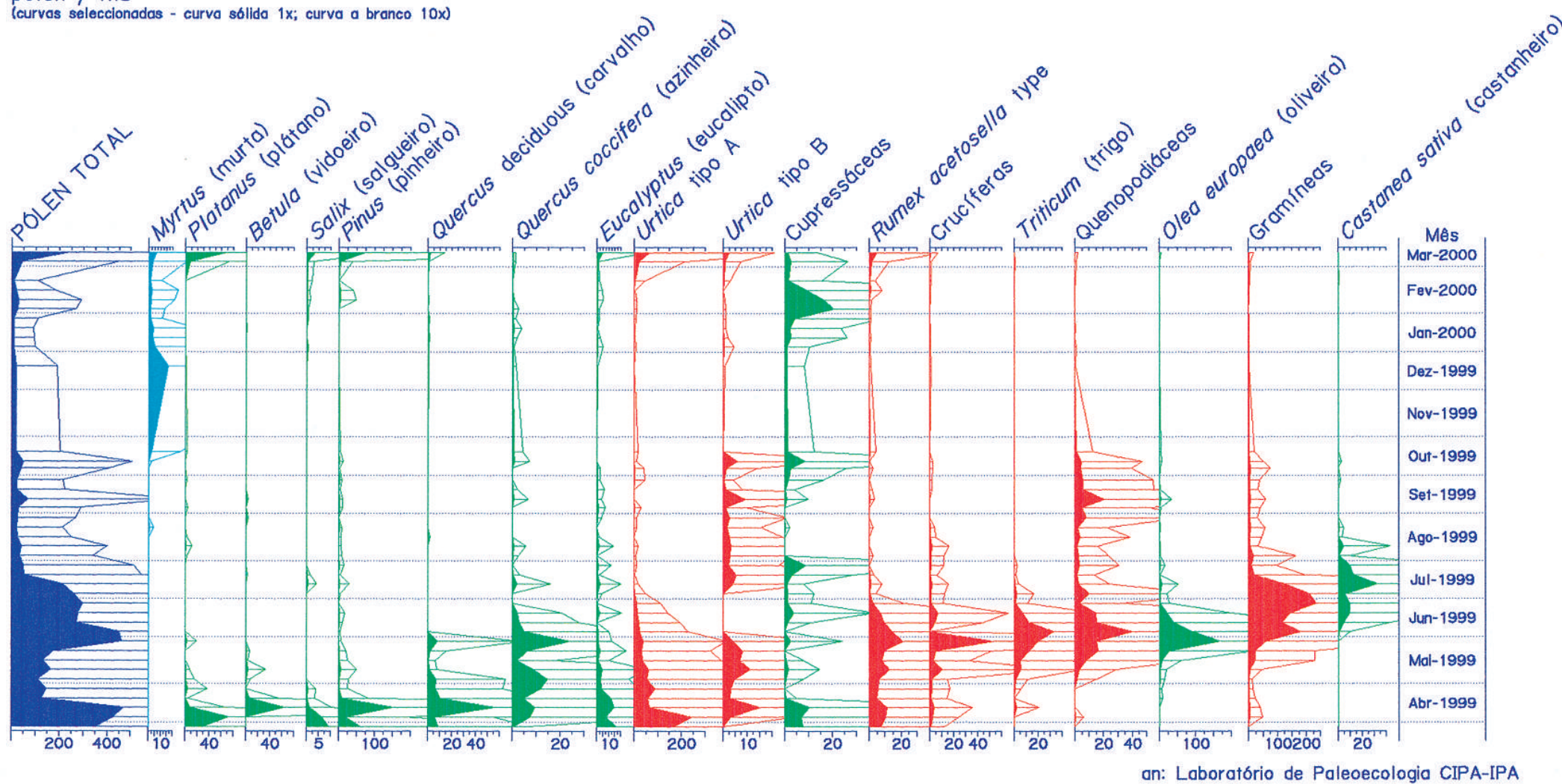
CALDAS DA RAINHA - 1999 CONCENTRAÇÃO POLÍNICA ATMOSFÉRICA SEMANAL pólen / m 3 (curvas seleccionadas - curva sólida 1x; curva a branco 10x)
